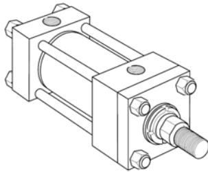
F 方式 侧面螺纹孔安装 (NFPA MS4 方式)
