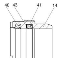
Gland 插装件和密封组件
