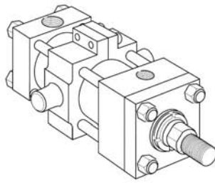
DD 方式 中间固定耳轴 (NFPA MT4 方式)
