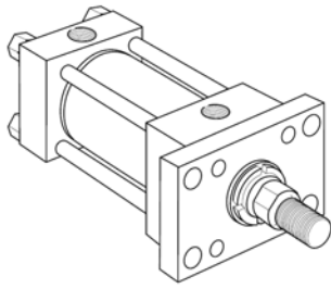
J 方式 缸头矩形法兰 (NFA MF1方式)
