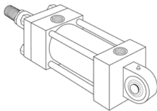
SBa 方式 球面轴承 (ISO 6982 和 CETOP RP88H)
