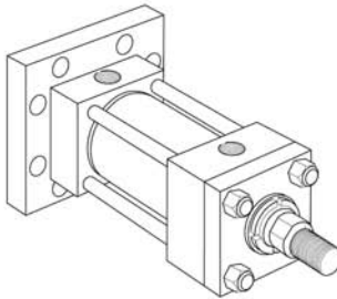
HB 方式 缸盖方形法兰 (NFA MF6 方式)
