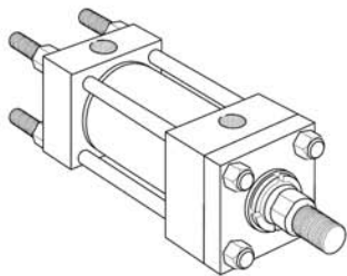
TC方式 缸盖端拉杆伸出 (NFA MX2 方式)
