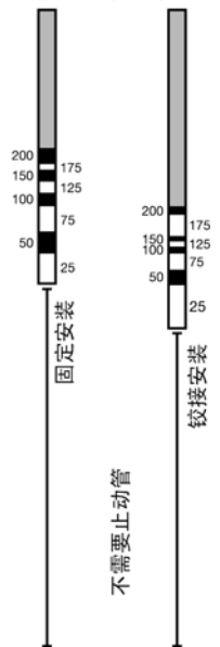
推荐的止动管长度 (mm)
