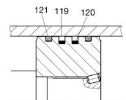
高负载活塞
