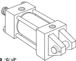
BB 方式 缸盖固定双耳环 (NFA MP1 方式)
