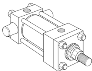
DB 方式 缸盖端耳轴 (NFA MT2 方式)
