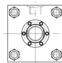
内径254mm (10") 液压缸 4 个拉杆结构形式
