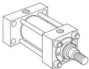
HH 方式 矩形缸盖 (NFA ME6 方式)
