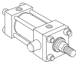
D 方式 缸头端耳轴 (NFA MT1 方式)
