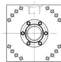
内径304.8mm (12") 液压缸 16 个拉杆结构形式
