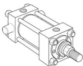
DB 方式 缸盖端耳轴 (NFA MT2 方式)
