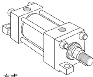
G 方式 端侧面凸耳 (NFPA MS7 方式)
