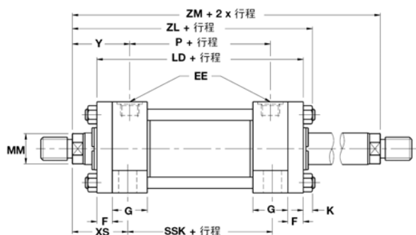
双活塞杆缸 缸内径38.1至203.2mm TB、TD、J、JB、JJ、C、 F、D、DD和G方式有货
