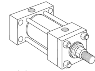
HH 方式 矩形缸盖 (NFPA ME6 方式)
