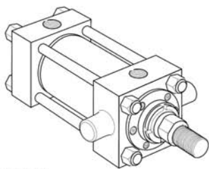
D 方式 缸头端耳轴 (NFA MT1 方式)
