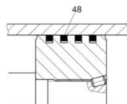
铸铁环活塞
