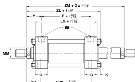
双活塞杆缸 缸内径254至304.8mm J、JB、JJ、C、D和DD有货
